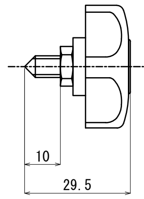
固定ノブ
