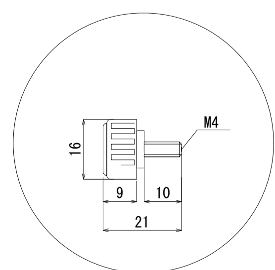
M4 ストッパーリング
