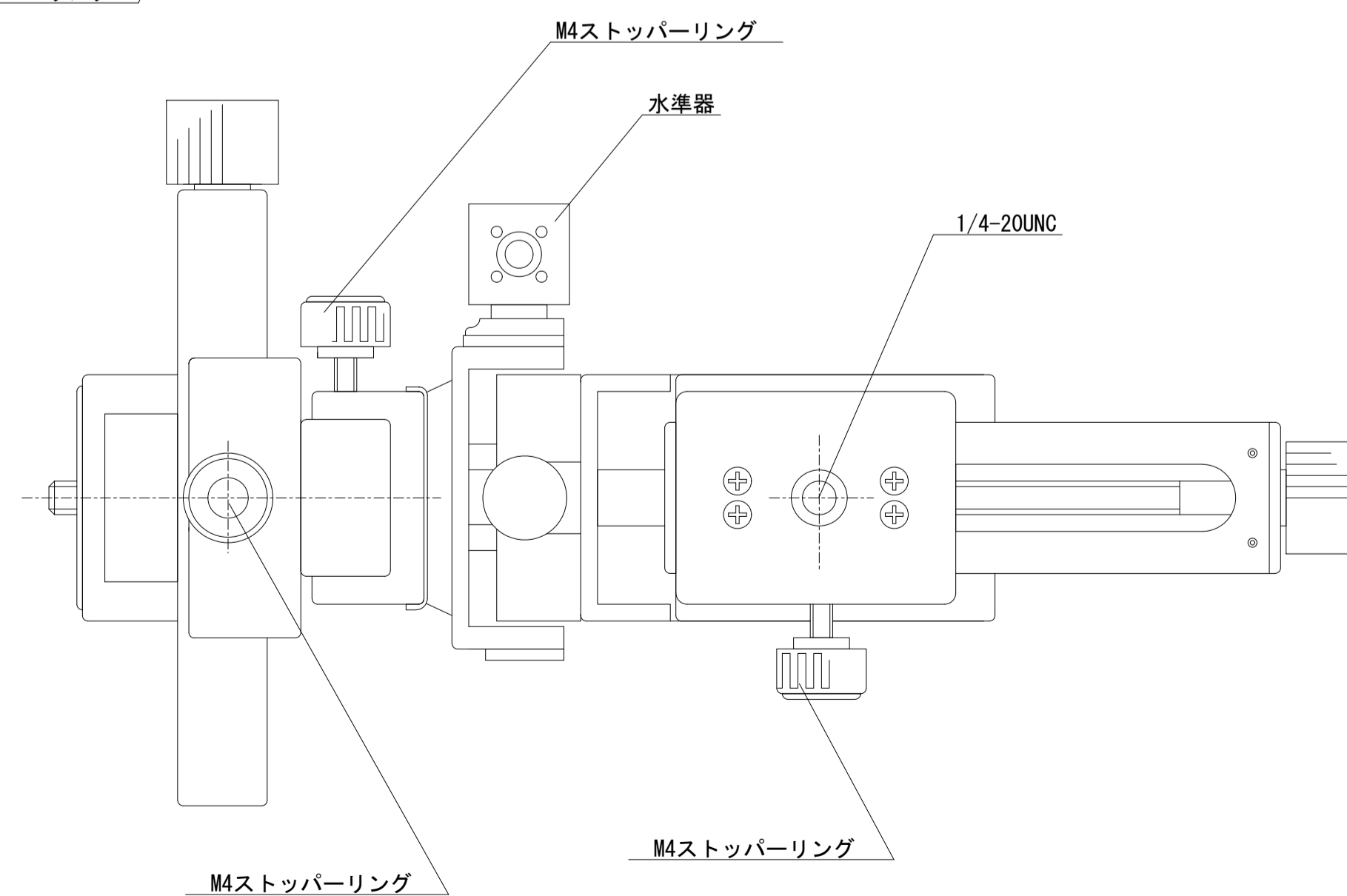
品名 : XYZ-L 微動装置 (ストッパー付き)
