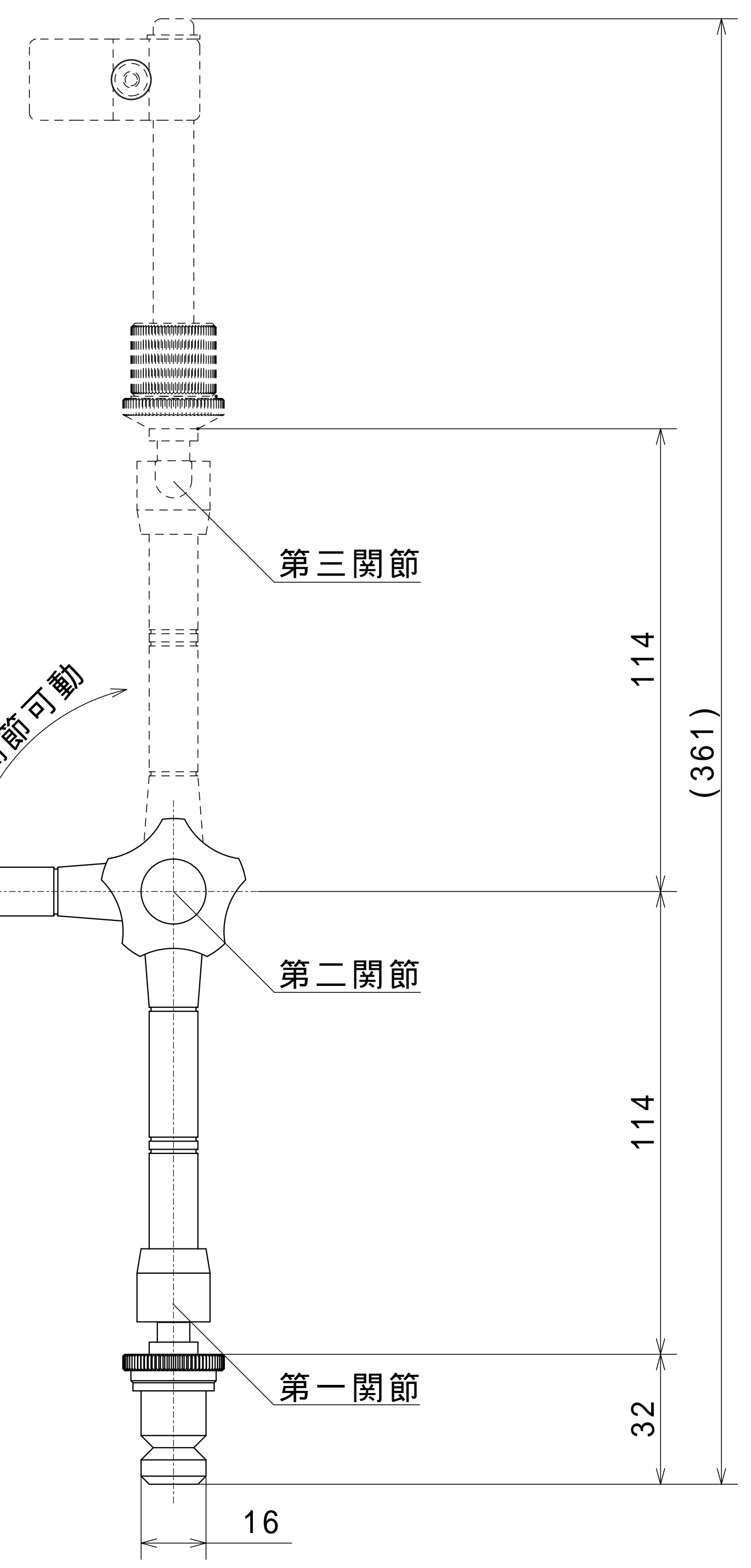
フレキシブルアーム(EX)ロングタイプ
