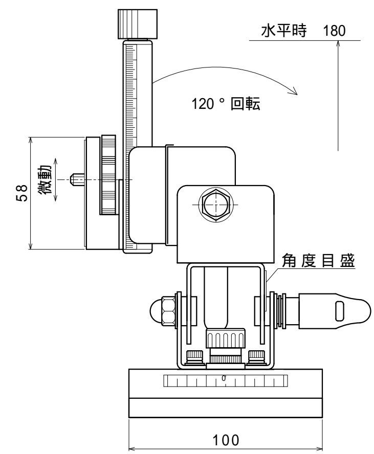
品名：ラインセンサカメラホルダー
