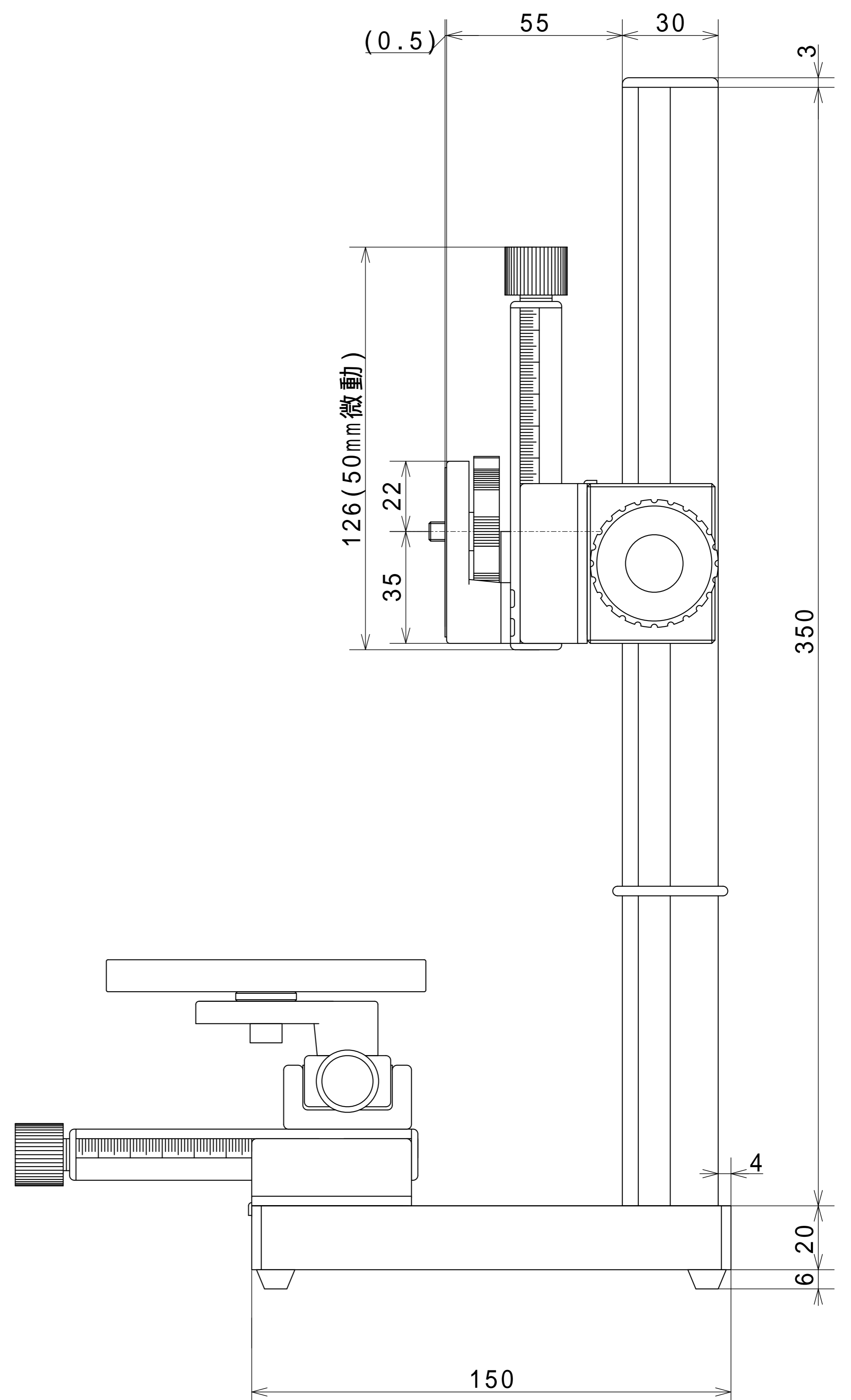
マイクロスタンドMK-2(350) XY ステージ
