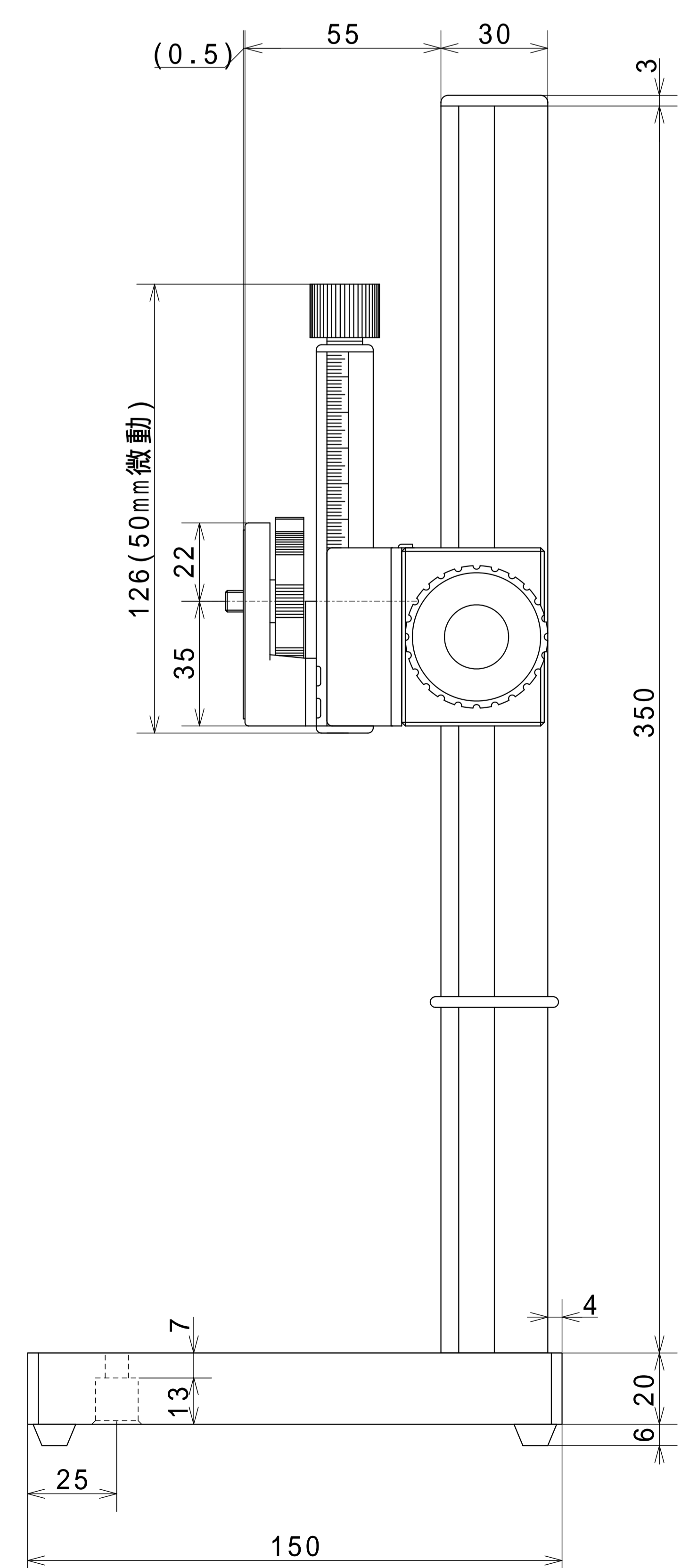
マイクロスタンド MK-2(350)
