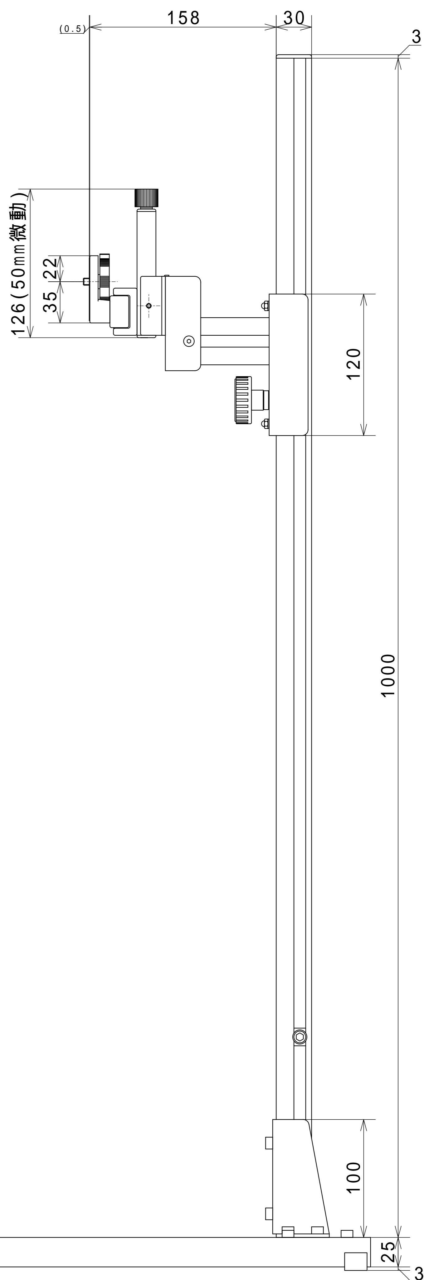
カメラスタンド SL(1000)
