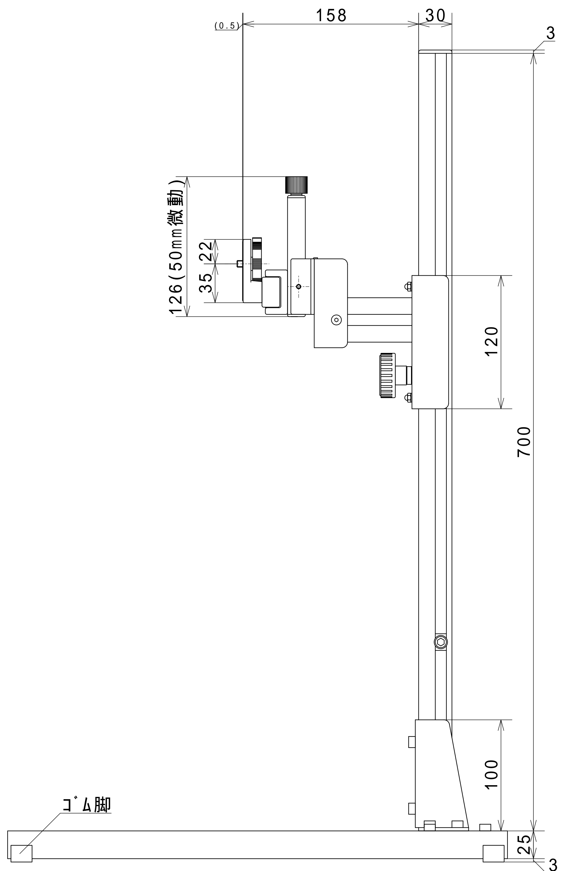
カメラスタンド SL(700)
